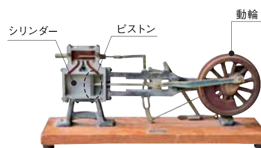
SLを動かす仕組みを表した模型。ボイラー内で発生した蒸気（現在は空気）がシリンダーへと送られ、中のピストンが左右に動くことで蒸気を送り出し動輪が動く
